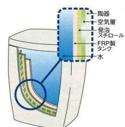
防露タンク断面
